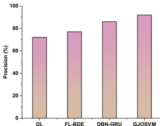
Fig. 4. Precision
